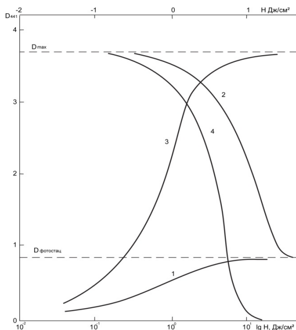
Рис.3. Характерные кривые окрашивания (1,3) и обесцвечивания (2,4) 6-Ф-5, 12-НХ на длинах волн облучения: 1 – обл.=441,2 нм (Робл.=1,5 мВт/см 2 ), 2 – обл.=441,2 нм (Робл.=1,5 мВт/см 2 ), 3 – обл.=320–410 нм (лампа ДРШ-250+светофильтр ФС-7; Робл.=10 мВт/см 2 ), 4 – обл.=480 нм (Робл.=1,0 мВт/см 2 ).
