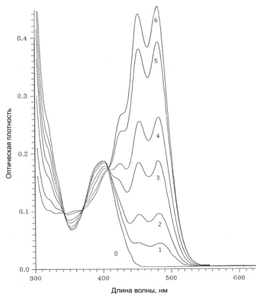
Рис.2. Спектры поглощения 6-Ф-5,12-НХ в толуоле: 0 – исходный раствор с преобладанием пара-хиноидной структуры (I); 1–6 – после облучения через интерференционный светофильтр с максимумом пропускания 400 нм (Робл.=0,33 мВт/см 2 ). Времена облучения: 15; 45; 105; 240; 480; и 980 с, соответственно.
