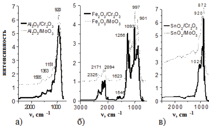
Рис. 1. ИК-спектры диффузного отражения смешанных оксидов на основе оксидов алюминия (а), железа (б) и олова (в)
